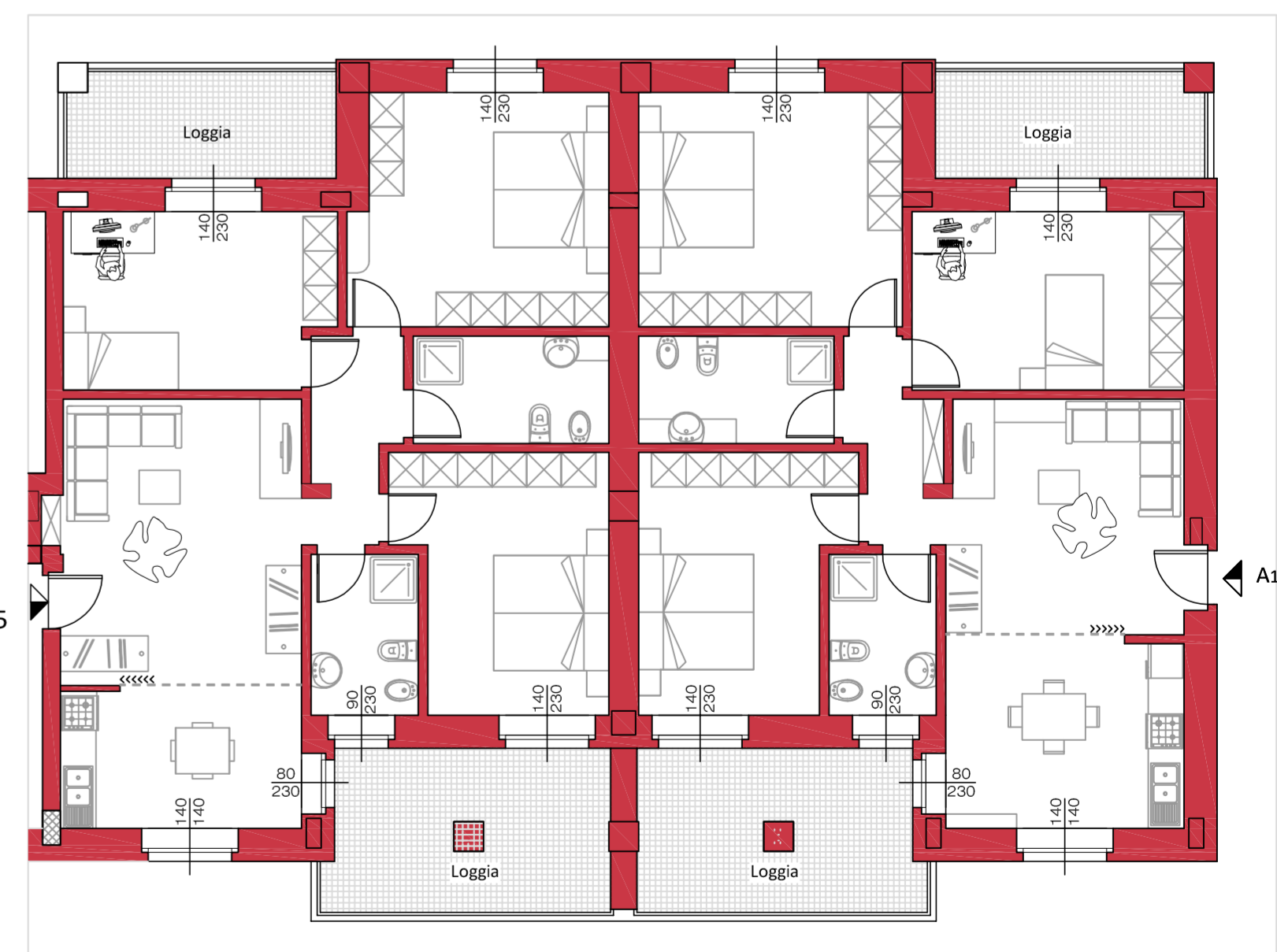
Soluzione alloggio B5 unico
